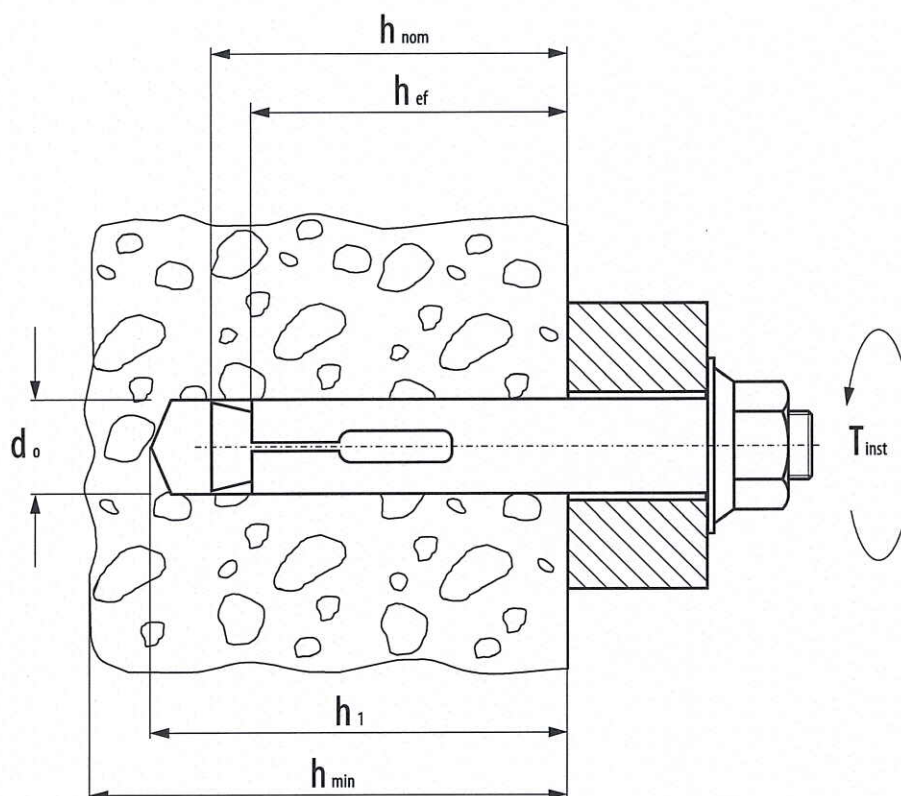
Rysunek B3. Parametry montażu stalowych łączników rozporowych ŁSI
