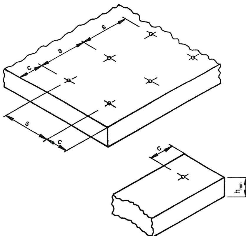
Rysunek B2. Parametry rozmieszczenia stalowych łączników rozporowych TRS w podłożu
